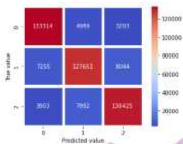
Gambar 4. 40 CM Porter Stemmer dan N-Gram Dataset 3
