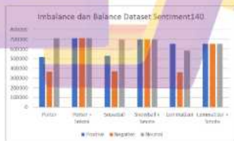
Gambar 4. 6 Grafik Imbalance dan Balance Dataset 3
