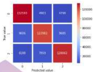
Gambar 4. 41 CM Porter Stemmer dan BoW Dataset 3
