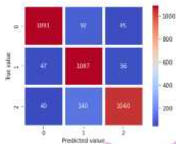
Gambar 4. 34 CM Porter Stemmer dan N-Gram Dataset 2
