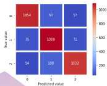
Gambar 4. 35 CM Porter Stemmer dan BoW Dataset 2
