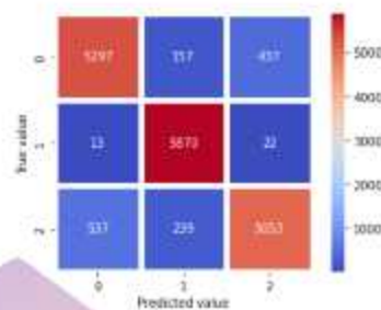
Gambar 4. 29 CM Porter Stemmer dan BoW Dataset 1
