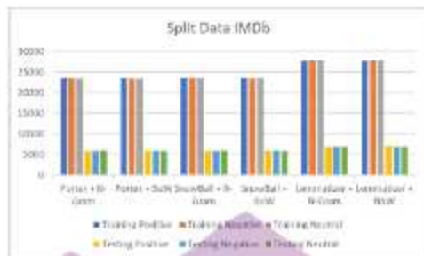
Gambar 4. 7 Grafik Split Data Dataset 1
